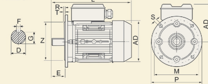
IMB5
