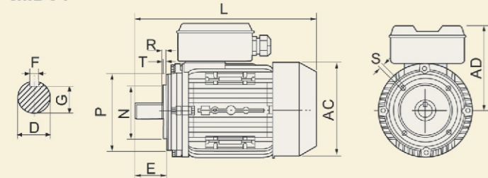
IMB14
